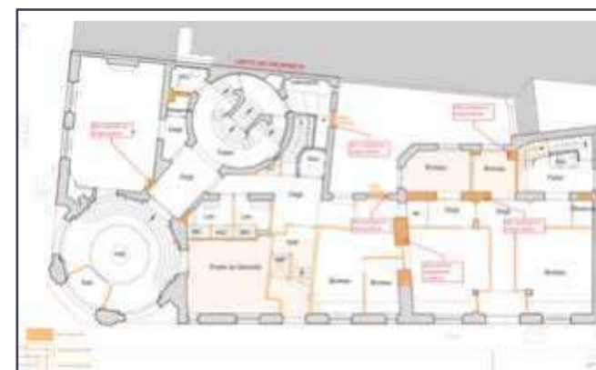
Plan des démolitions envisagées au rez-de-chaussée (© DVVD Architectes Ingénieurs).
