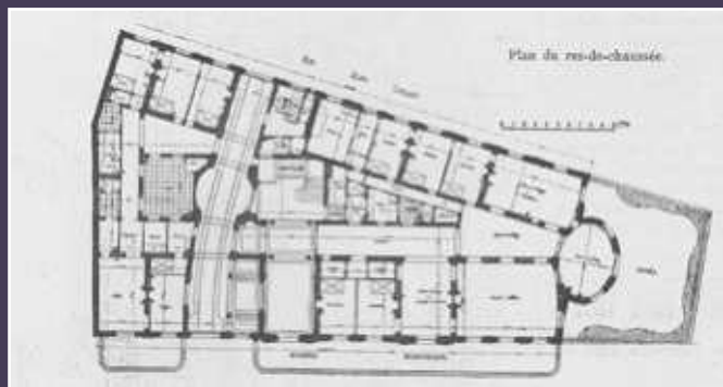
Plan du rez-de-chaussée, 1899 (publié dans L'Architecture , n° 5, 31 janvier 1903, p. 40).
