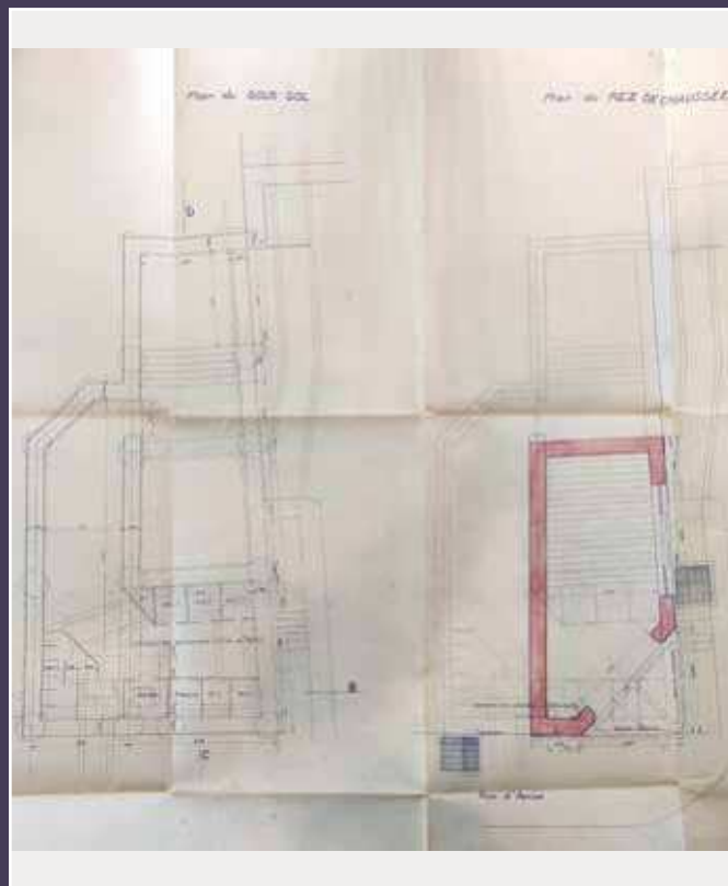
Plans du sous-sol et du rez-de-chaussée, 1932 (Archives de Paris).
