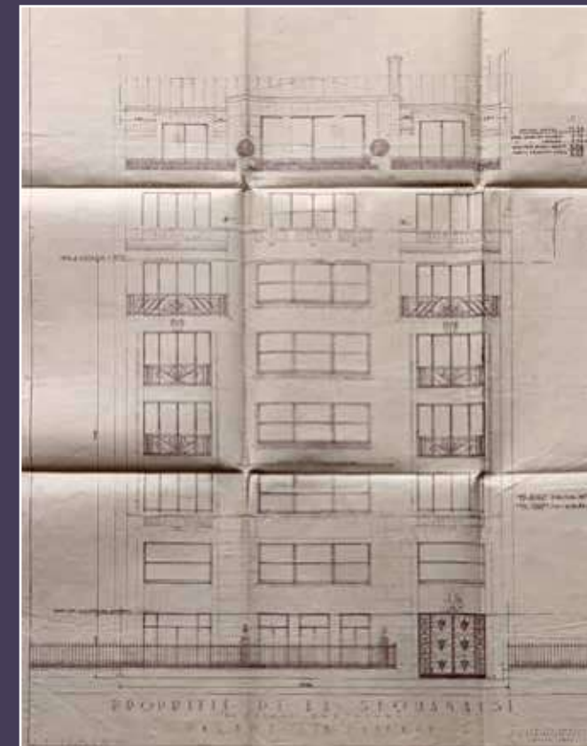
Élévation donnant sur l'avenue Montaigne, M. Julien et L. Duhayon, 1935 (Archives de Paris).
