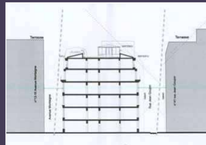
Coupe transversale, état projeté (© Agence Dary Architectes).
