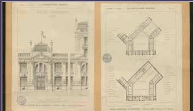
Planche issue du concours de 1896 pour la construction de l'ES-CP (publiée dans La Construction moderne , 1896) (BHVP).
