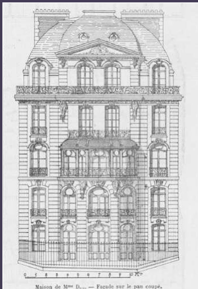
Élévation du pan coupé entre l'avenue Montaigne et la rue Jean Goujon, 1899 (publiée dans L'Architecture , n° 5, 31 janvier 1903, p.39).
