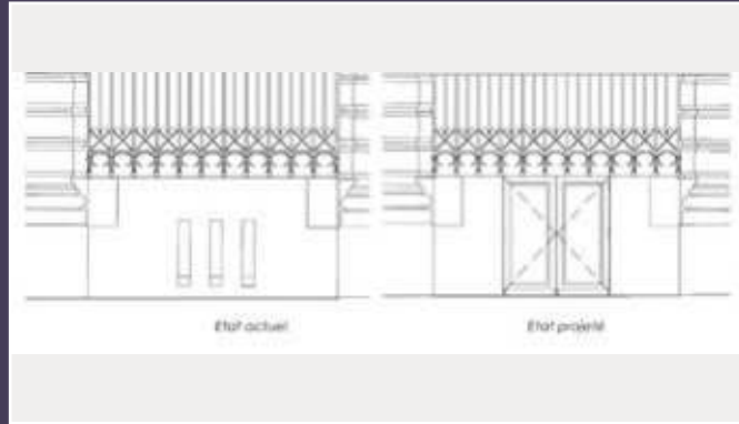
Détail du socle, état actuel (à gauche) et projet (à droite) (© Chiambaretta / Lagneau).
