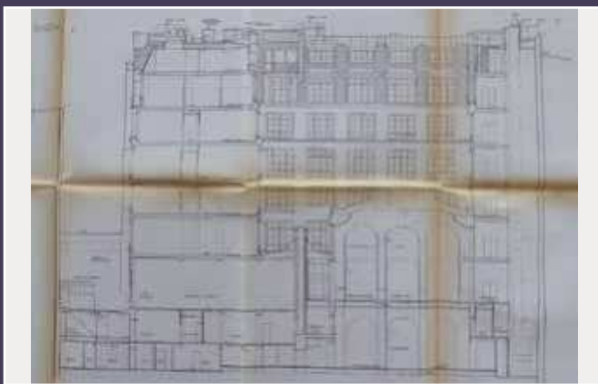
8-12, rue Boissy d'Anglas, coupe CC, 1997 (Archives de Paris).
