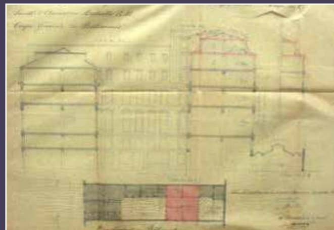
9, rue Royale, coupe générale des bâtiments et plan général des bâtiments, 1909 (Archives de Paris).
