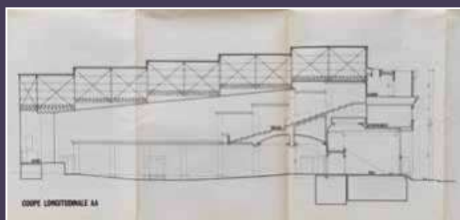
Coupe longitudinale, état existant en 1977 (Archives de Paris).
