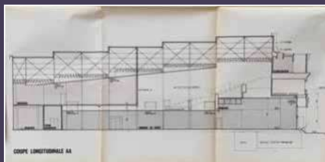
Coupe longitudinale, état projeté en 1977 (Archives de Paris).
