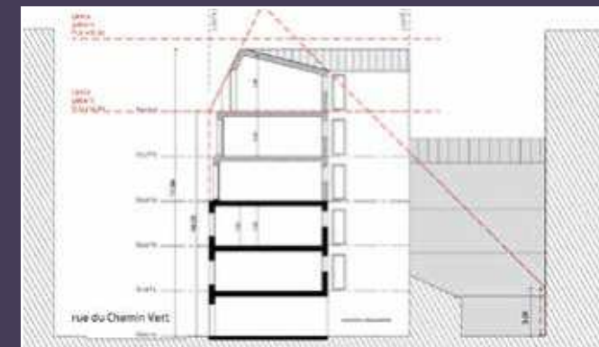
Coupe, état projeté. Projet présenté en novembre 2019 (© North by Northwest).
