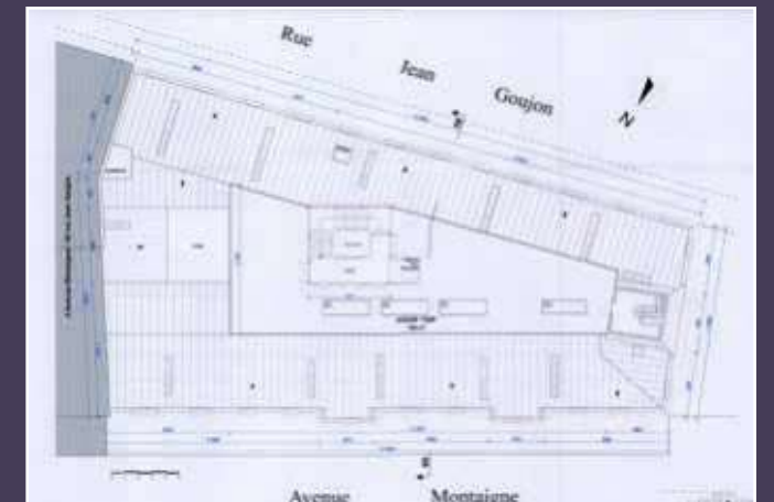
Plan des toitures, état projeté (© Agence Dary Architectes).
