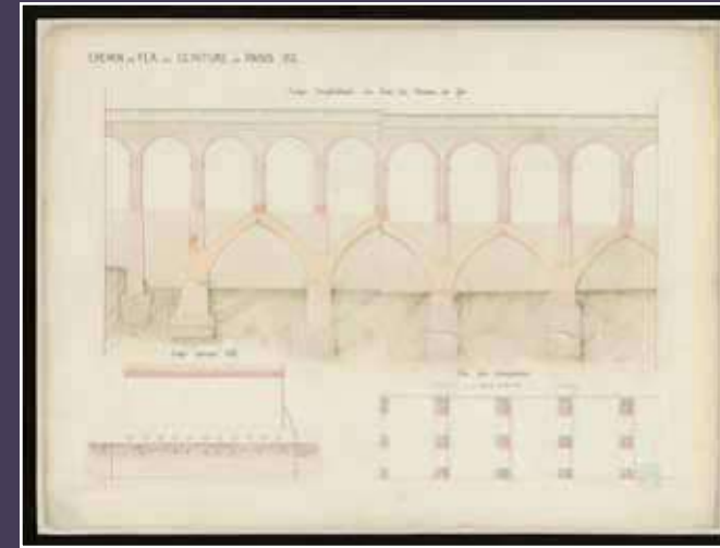
Petite Ceinture rive gauche, coupe longitudinale sur l'axe du chemin de fer et plan des maçonneries (BHVP).
