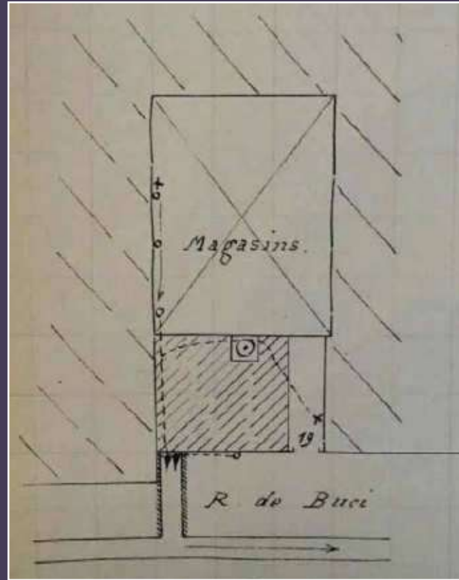
Fiche sanitaire de l'immeuble 19 rue de Buci. Schéma de l'implantation des corps de bâtiment. 1883 (Archives de Paris).
