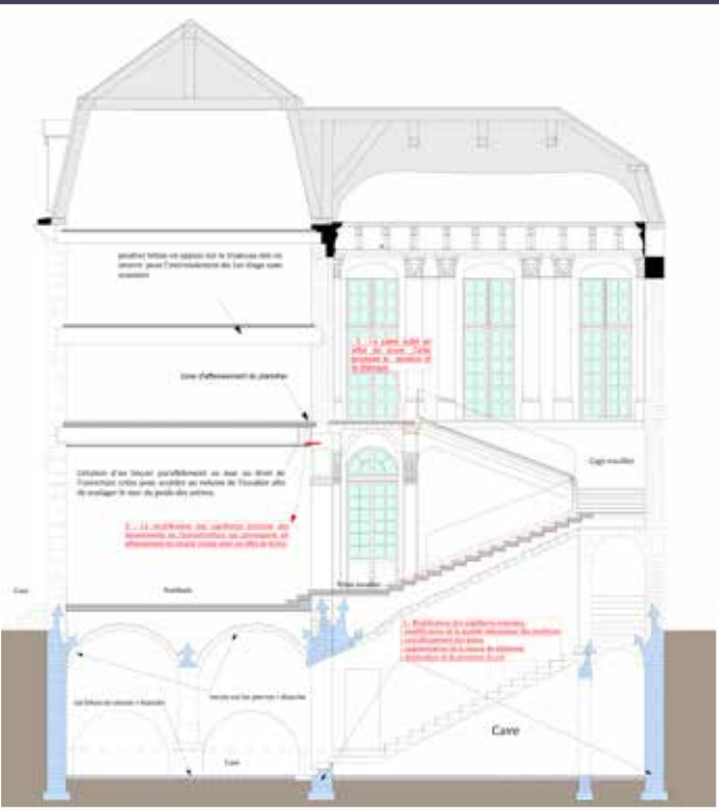
Coupe transversale de l'hôtel avec indication des désordres (© cabinet Jean Charpentier).
