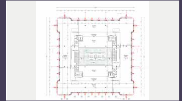
Plan du R+3, état projeté (© &Givry architectes).
