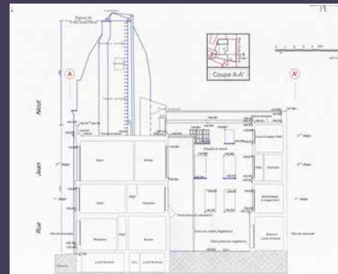
Coupe transversale, état existant (© Jean-Pierre Penin Architecte)
