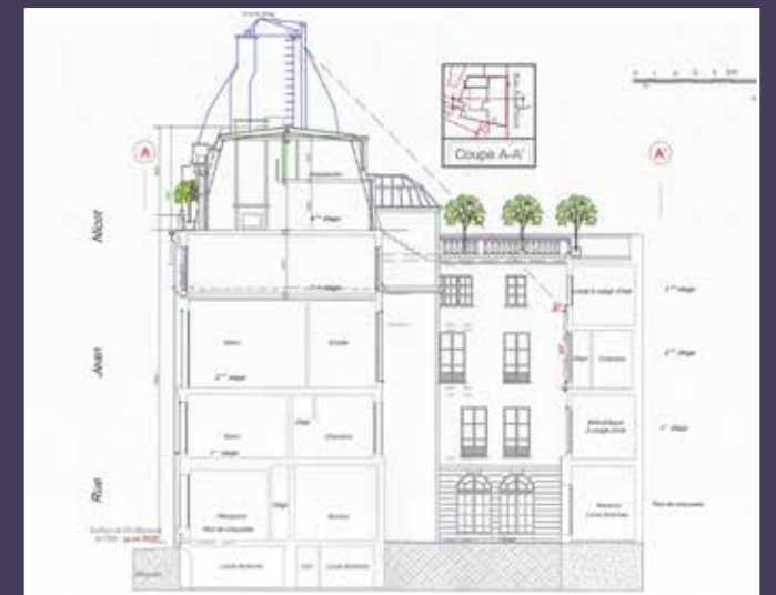
Coupe transversale, état projeté avec la surélévation (© Jean-Pierre Penin Architecte)
