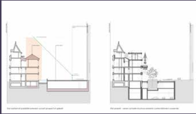
Coupe sur le double aile de la rue de l'Université, état actuel avec démolitions et état projeté (© COS architectes).
