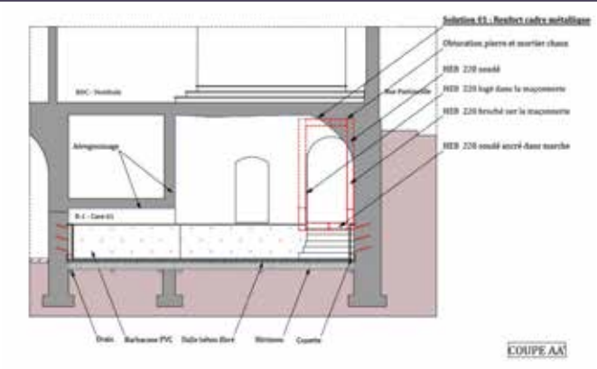
Solution 1 envisagée pour le mur de contreventement de la cave (cadre métallique) (© cabinet Jean Charpentier).
