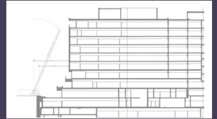
Coupe de l'existant illustrant la problématique de la sécurité incendie (© DTACC).
