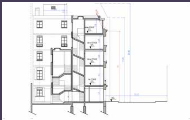
Coupe de l'immeuble passant sur les cages d'escaliers, état projeté (© Jean-Pierre Lesieur architecte).
