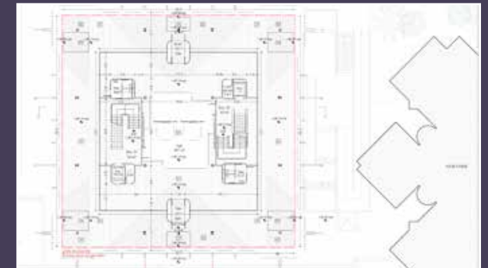
Plan du rez-de-dalle, état projeté (© &Givry architectes).
