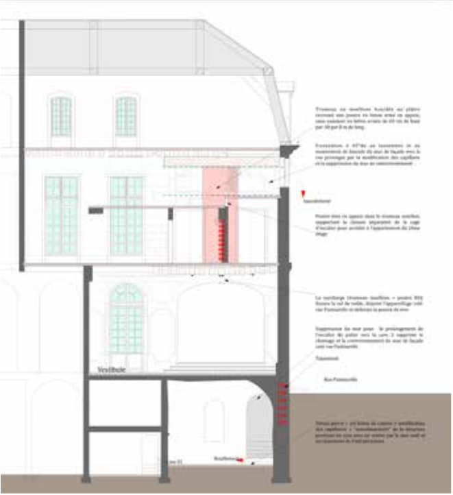
Coupe longitudinale de l'hôtel avec indication des désordres (© cabinet Jean Charpentier).
